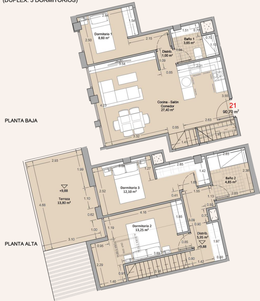
VIVIENDA 21 Sup.construida 97,18 m 2 (DÚPLEX. 3 DORMITORIOS)
