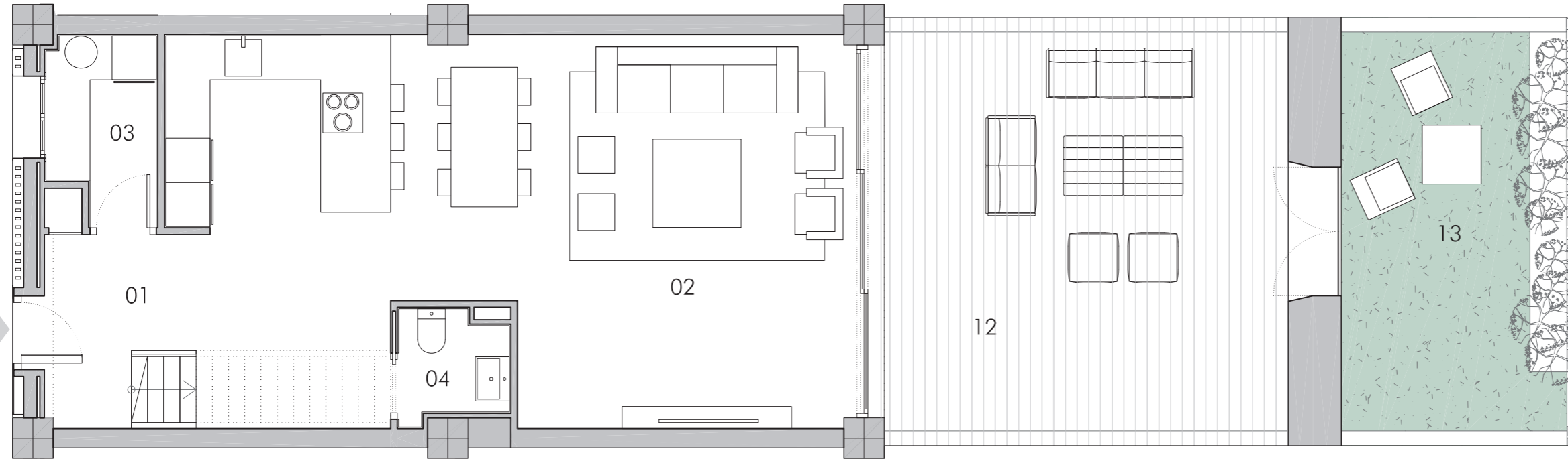
Planta baja
