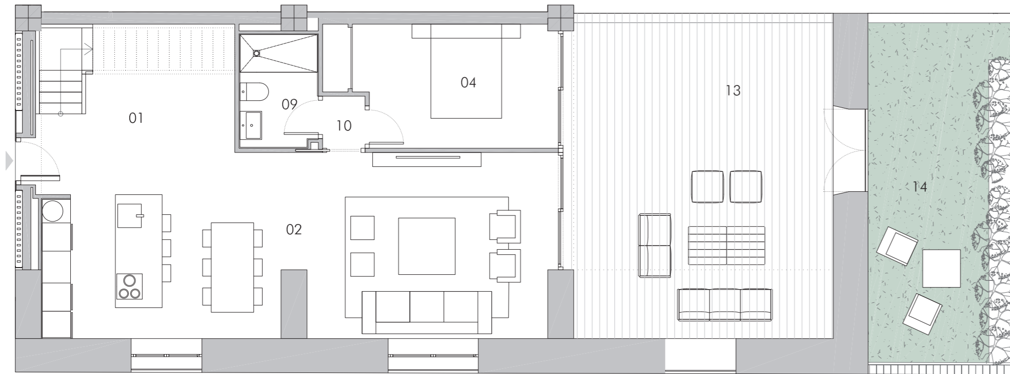
Planta baja
