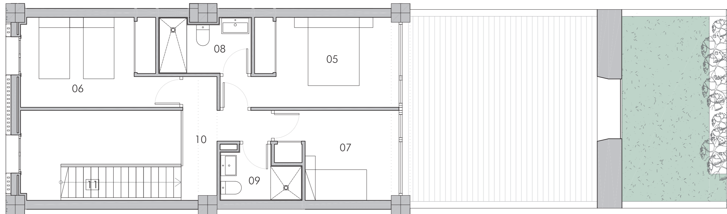
Planta primera
