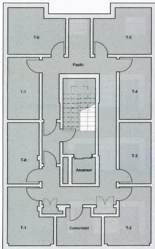
Planta Sótano
