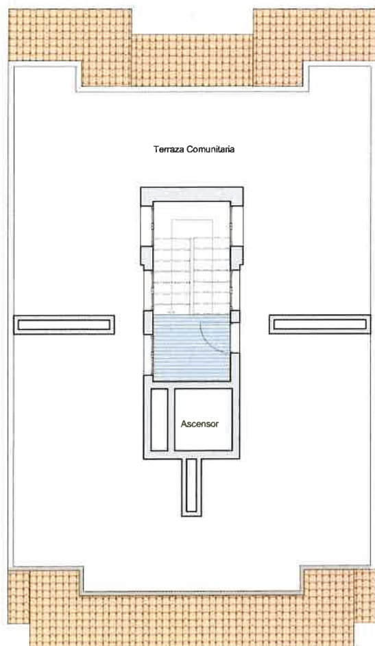
Planta Torreón
