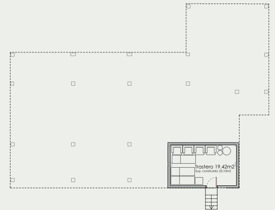
PLANTA SÓTANO
