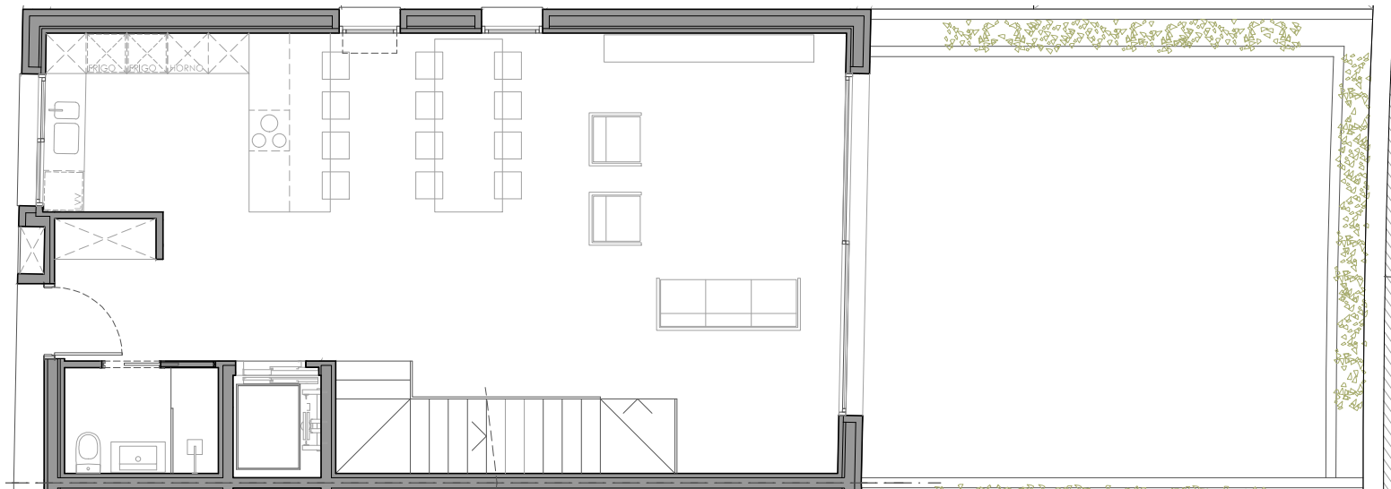
PLANTA BAJA
