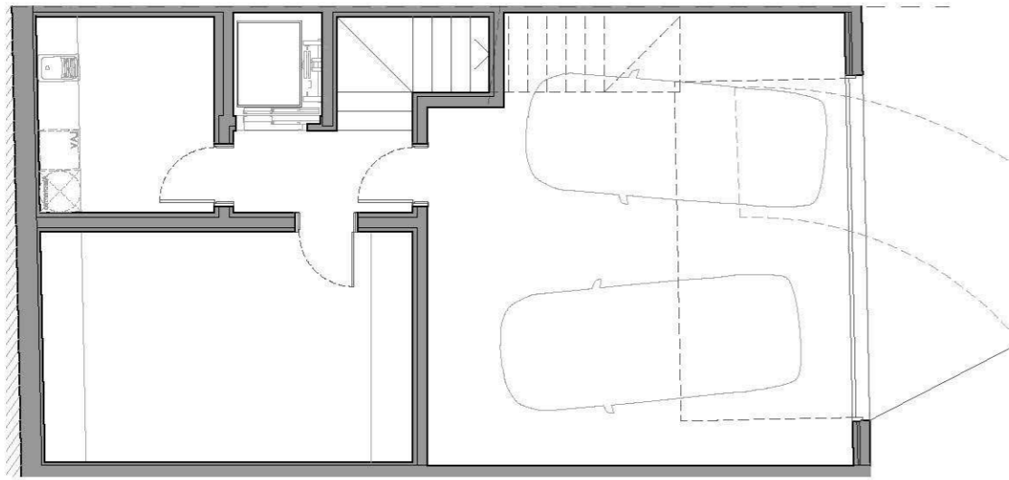
PLANTA SÓTANO
