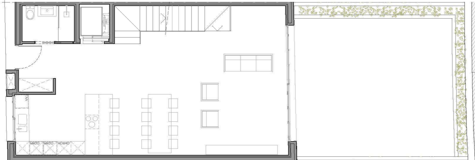
PLANTA BAJA
