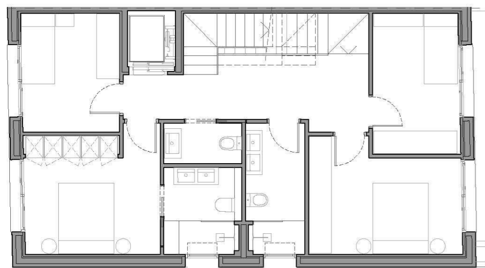
PLANTA PRIMERA
