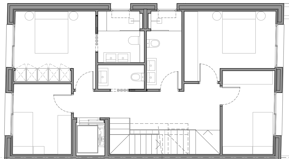
PLANTA PRIMERA
