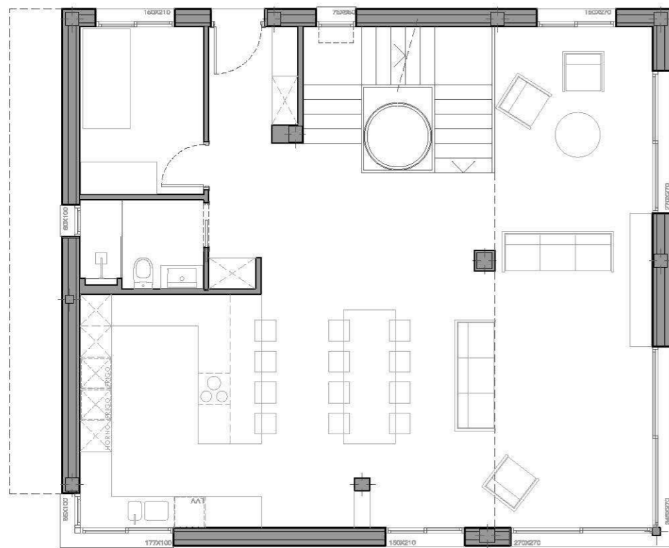
PLANTA BAJA
