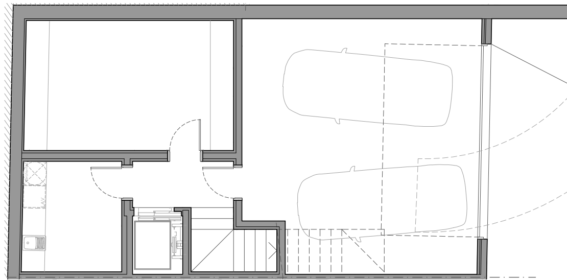
PLANTA SÓTANO
