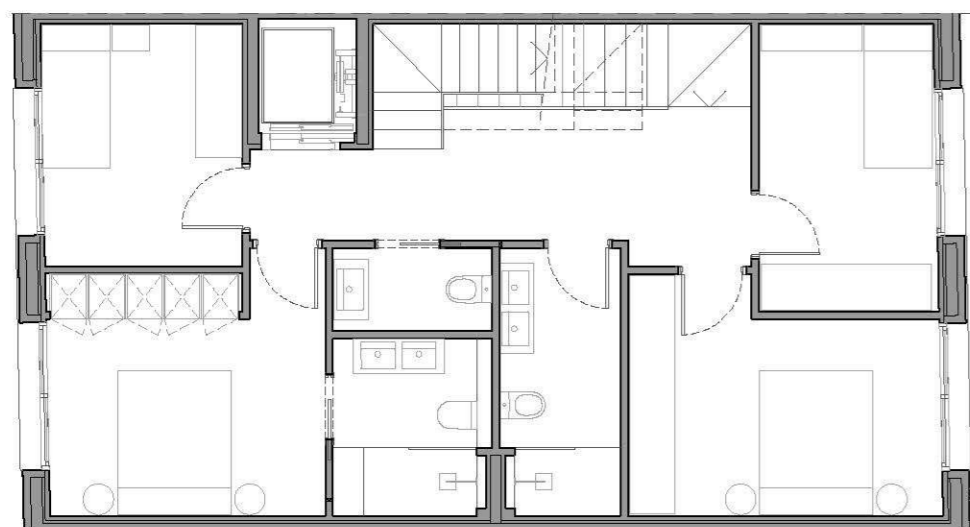
PLANTA PRIMERA
