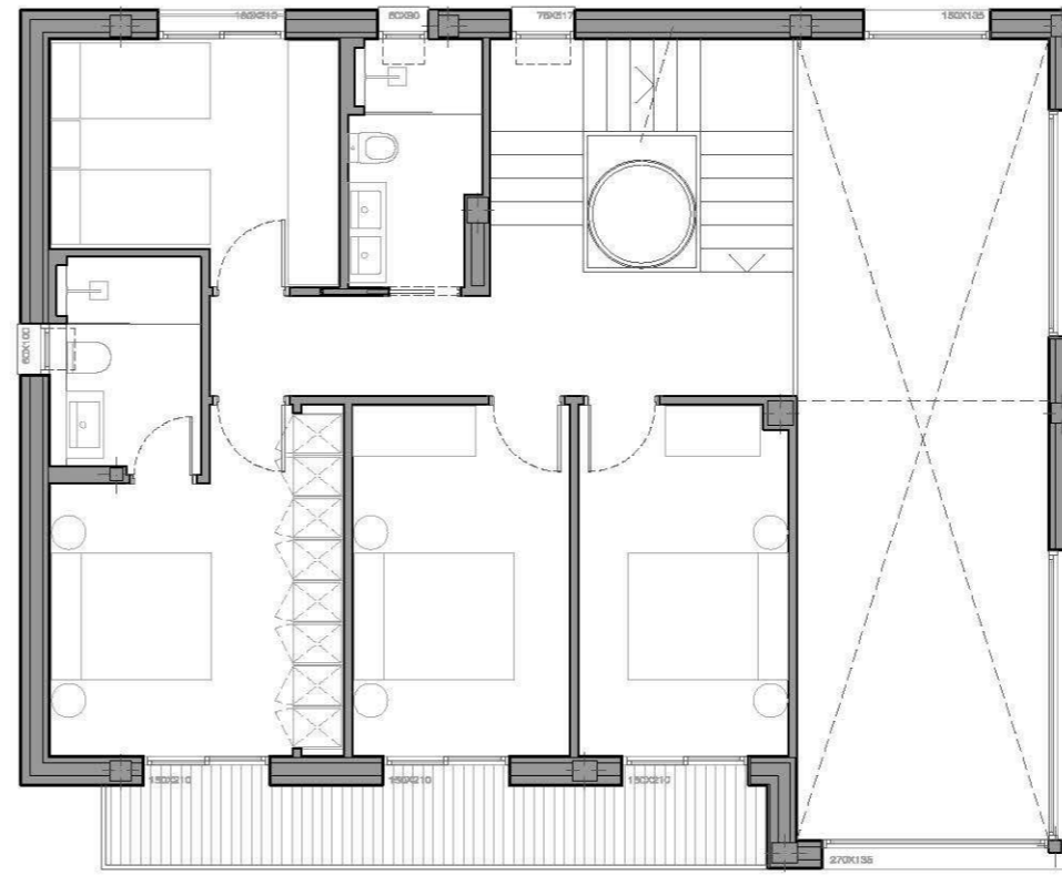
PLANTA PRIMERA
