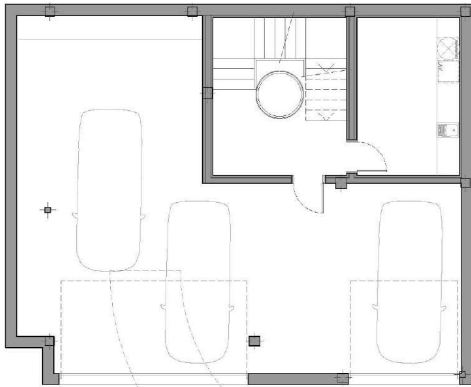
PLANTA SÓTANO
