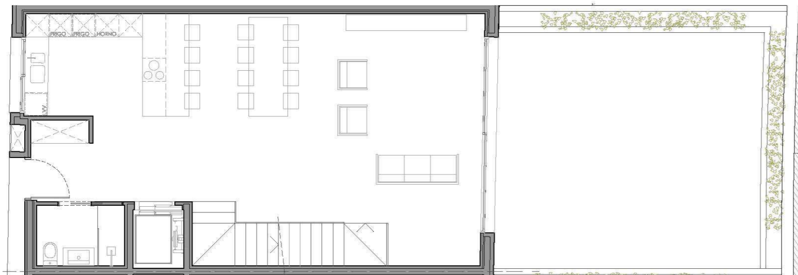
PLANTA BAJA
