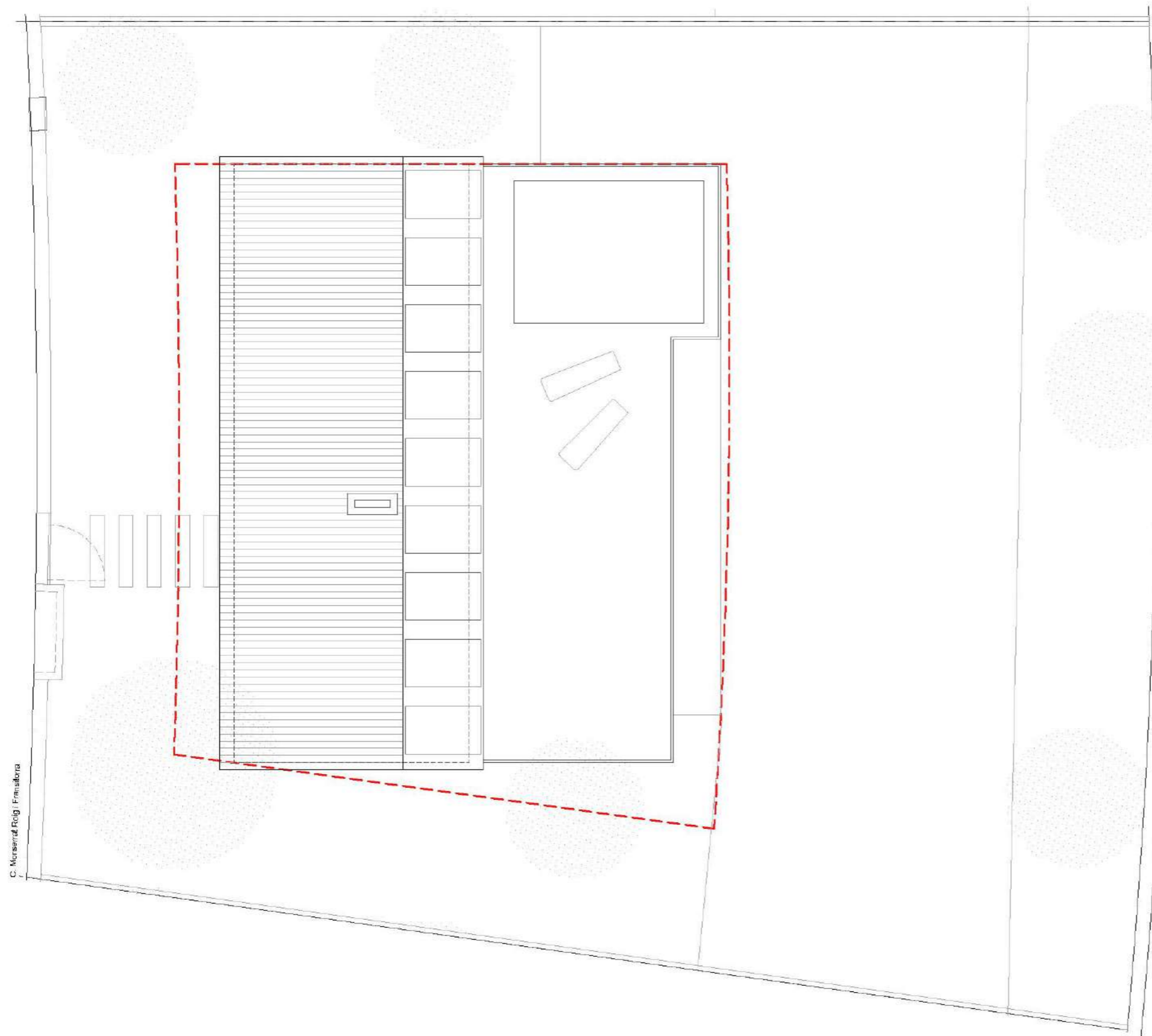
PLANTA CUBIERTA
