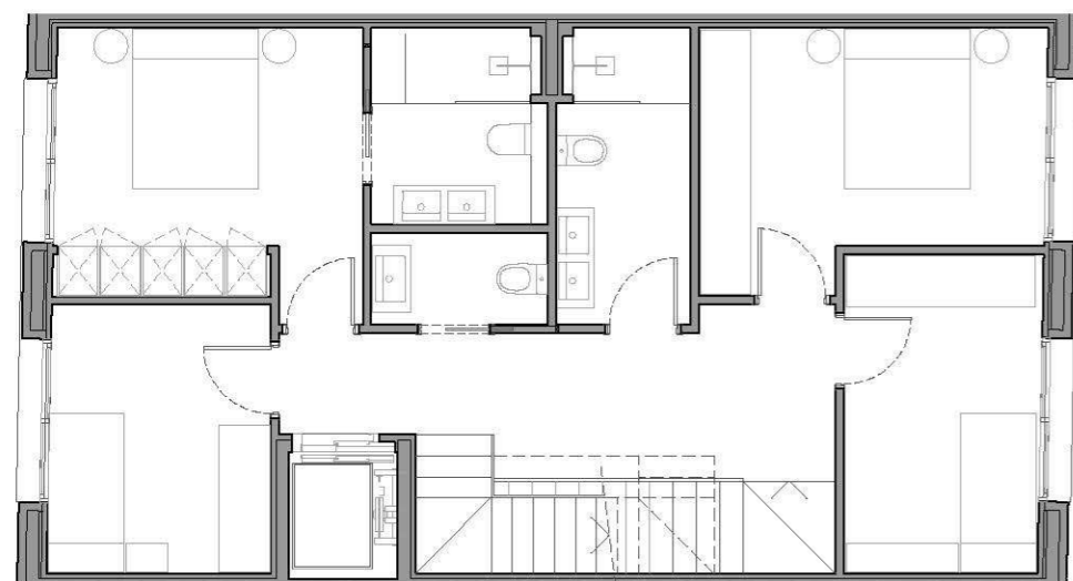
PLANTA PRIMERA
