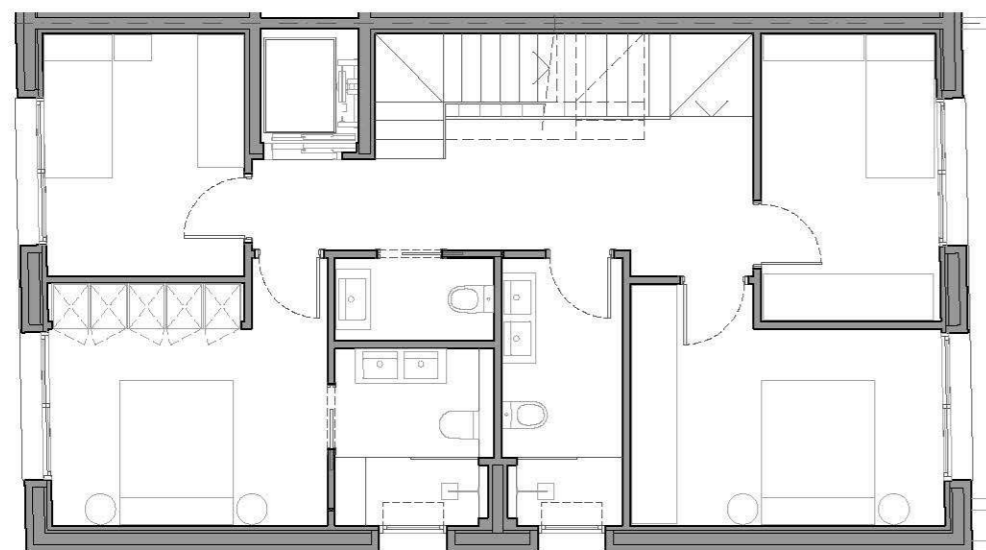
PLANTA PRIMERA
