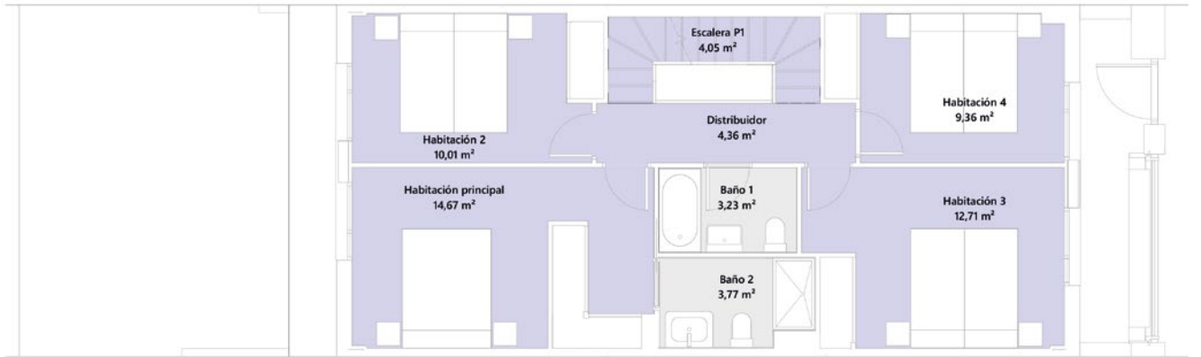
Planta Primera
