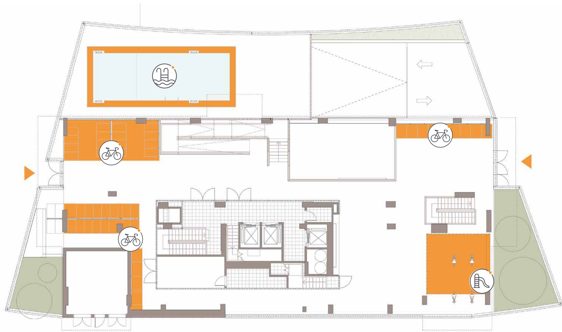
PLANTA BAJA
