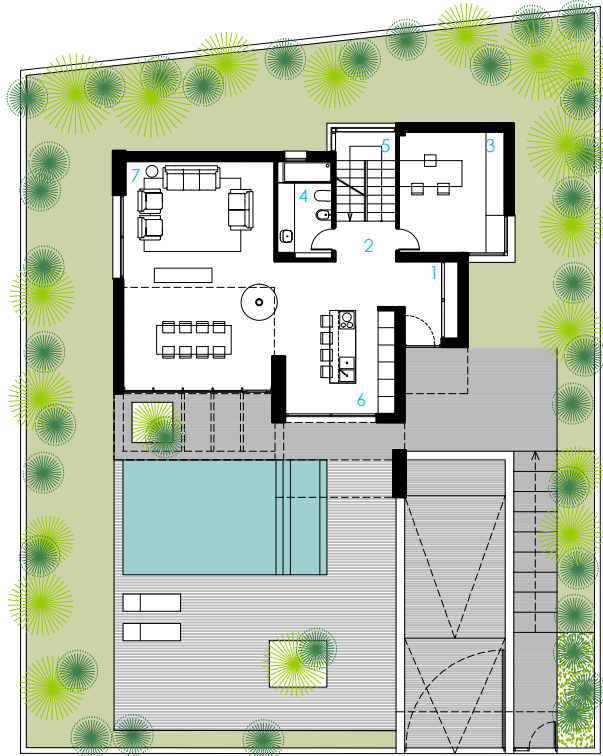
SUPERFICIES ÚTILES [m 2 ] - USEFUL SURFACE [m 2 ]
