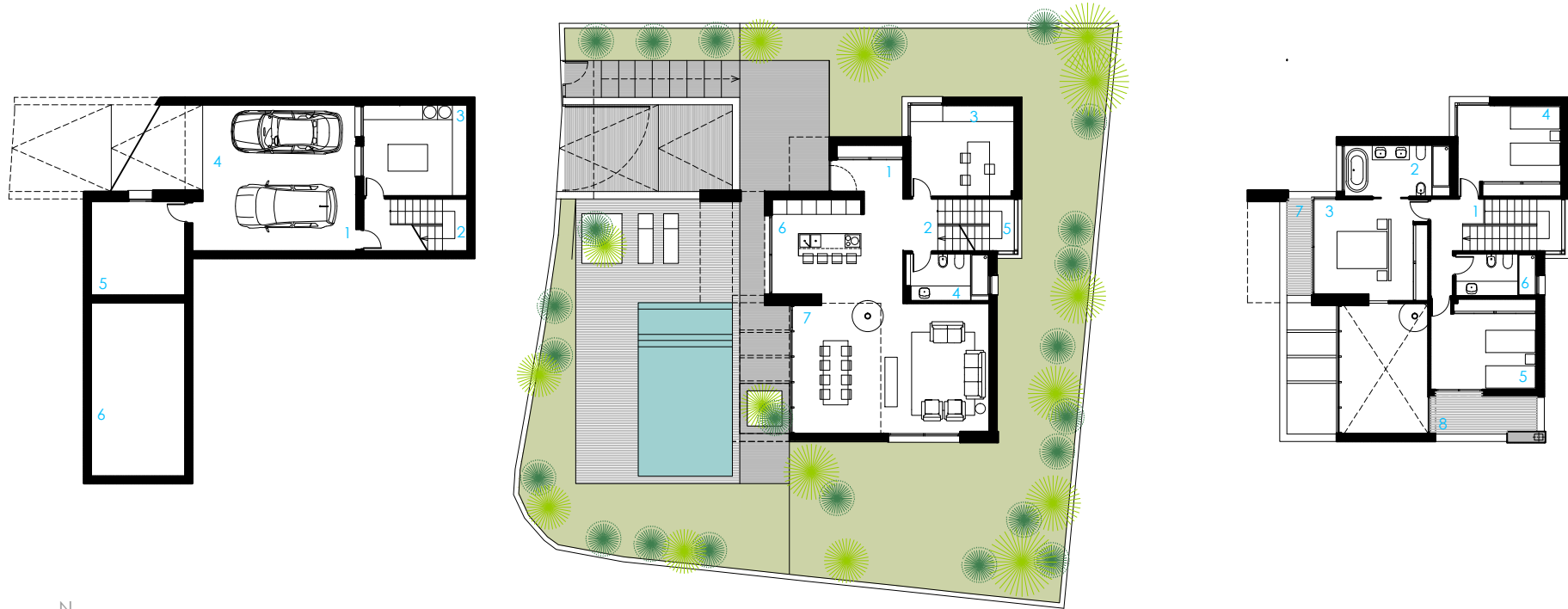
PLANTA SEMISÓTANO BASEMENT
