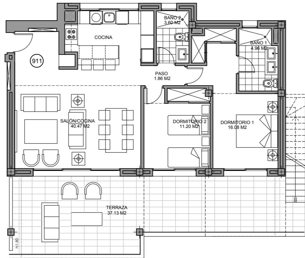
Planta Primera
