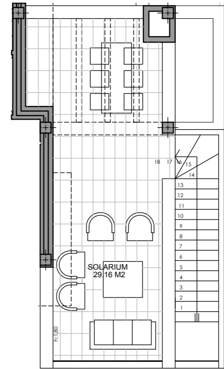
Planta Solarium
