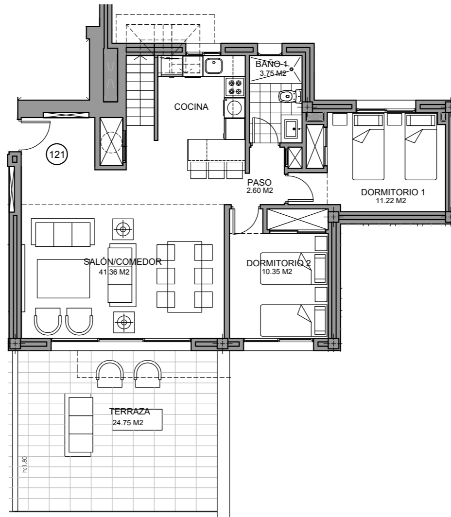
Planta Segunda
