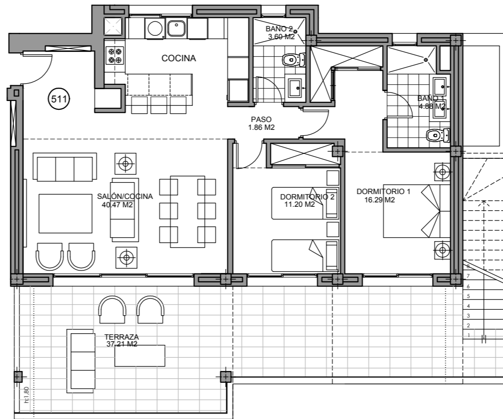
Planta Primera
