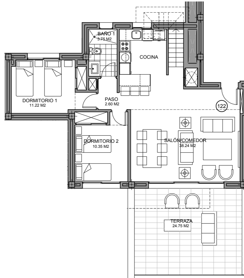
Planta Segunda
