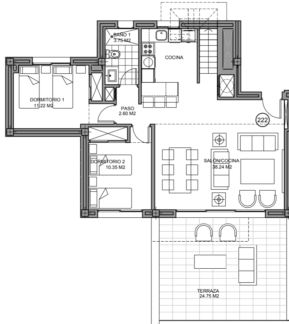
Planta Segunda
