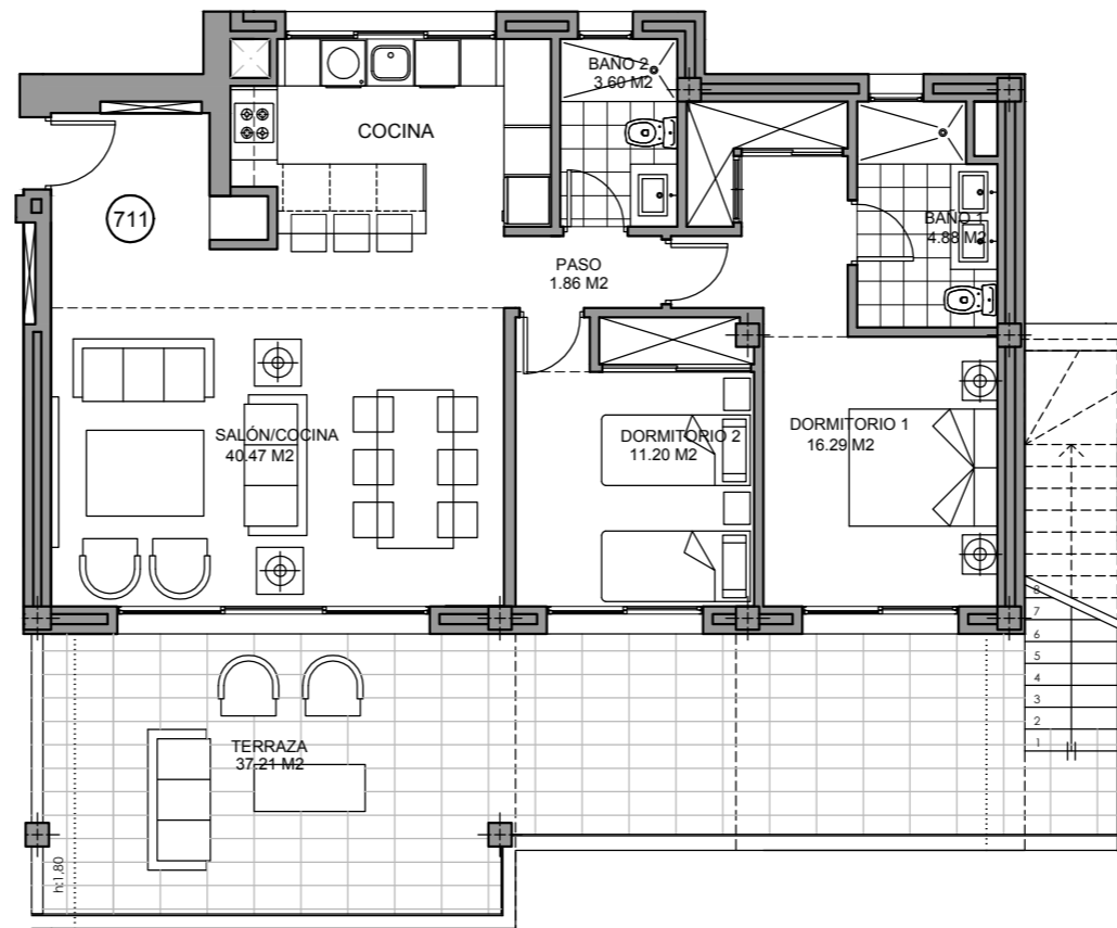
Planta Primera
