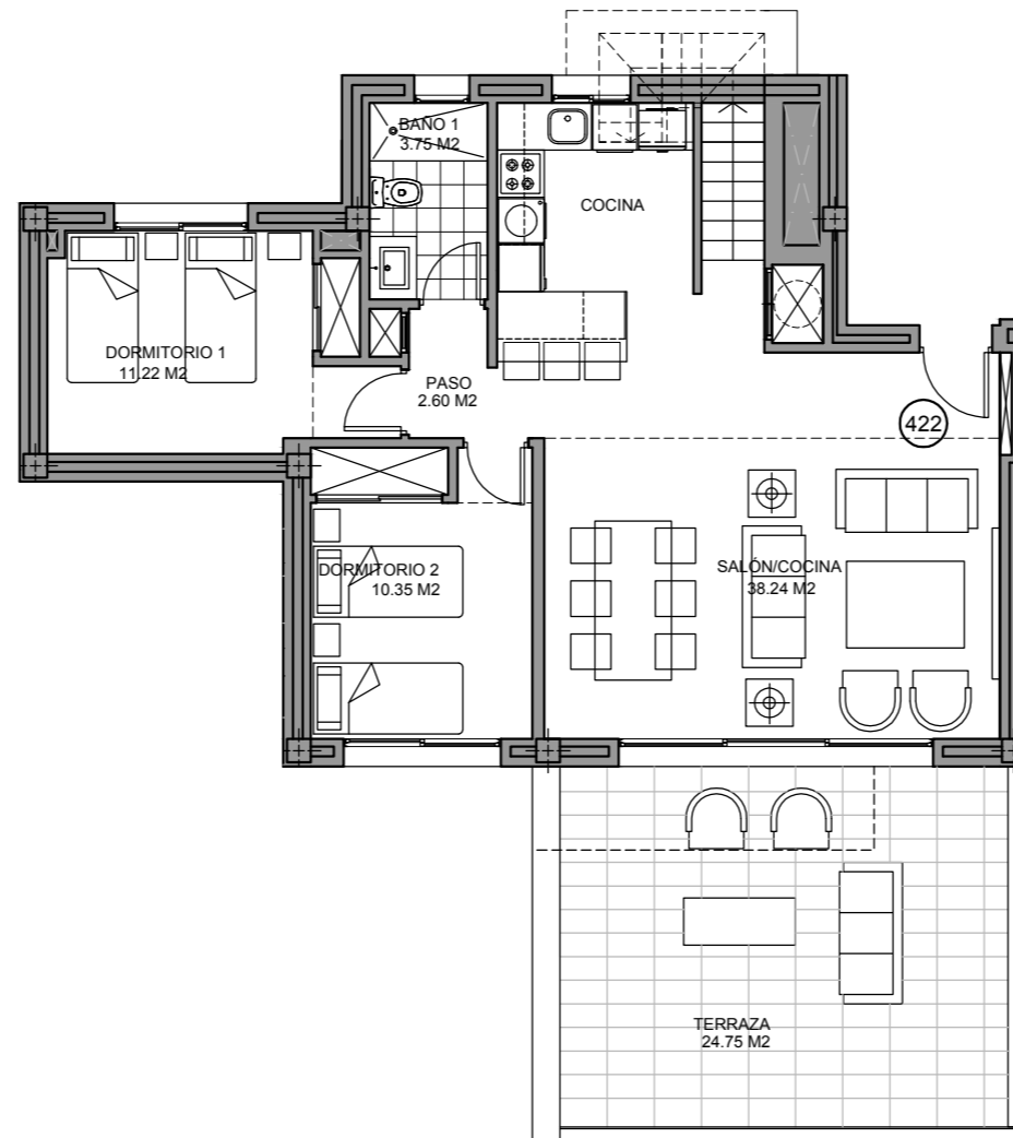
Planta Segunda
