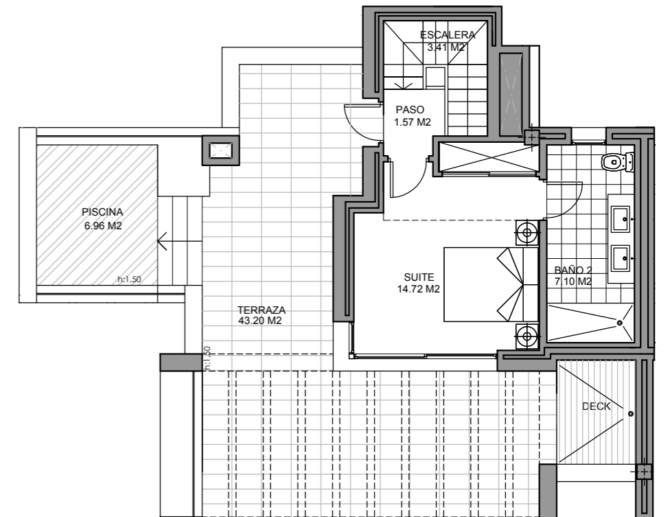
Planta Ático
