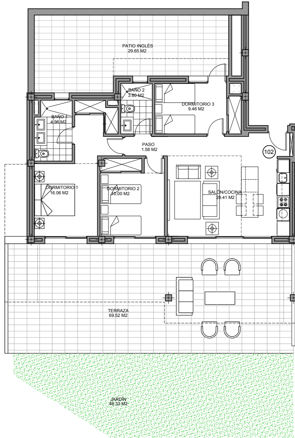
Planta Baja
