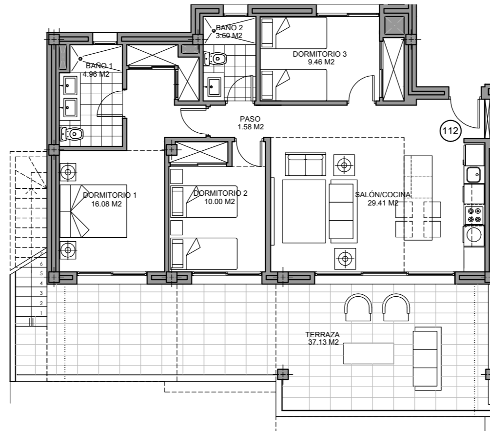
Planta Primera
