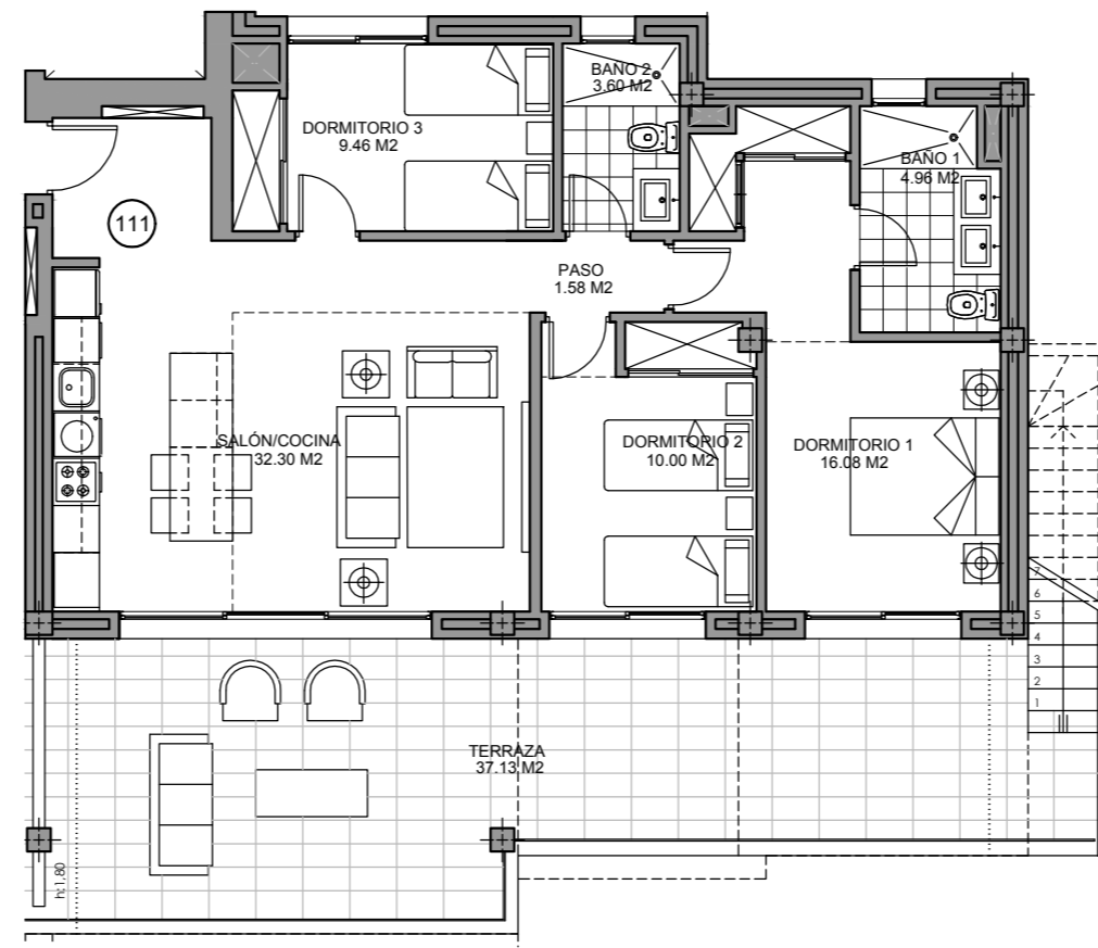
Planta Primera
