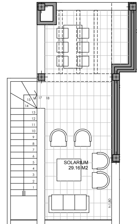
Planta Solarium
