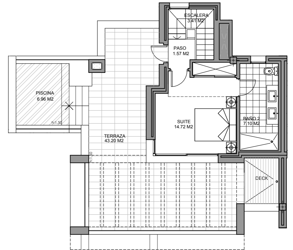
Planta Ático
