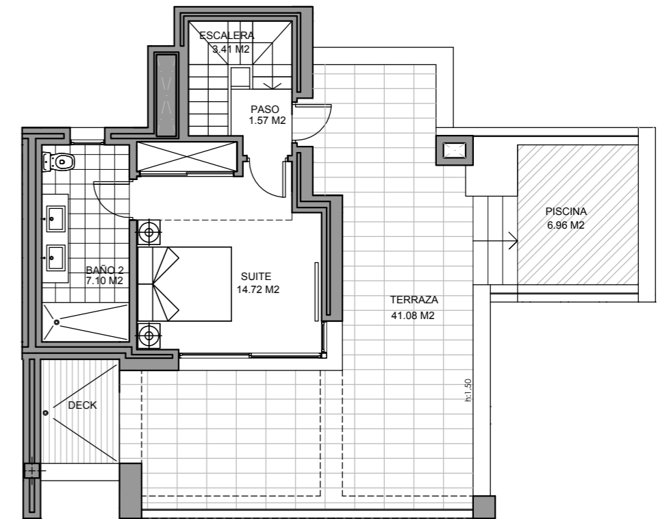
Planta Ático
