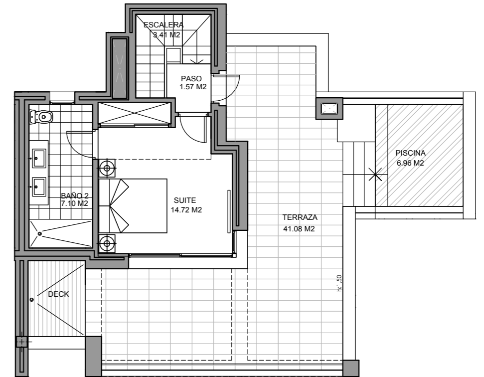
Planta Solarium
