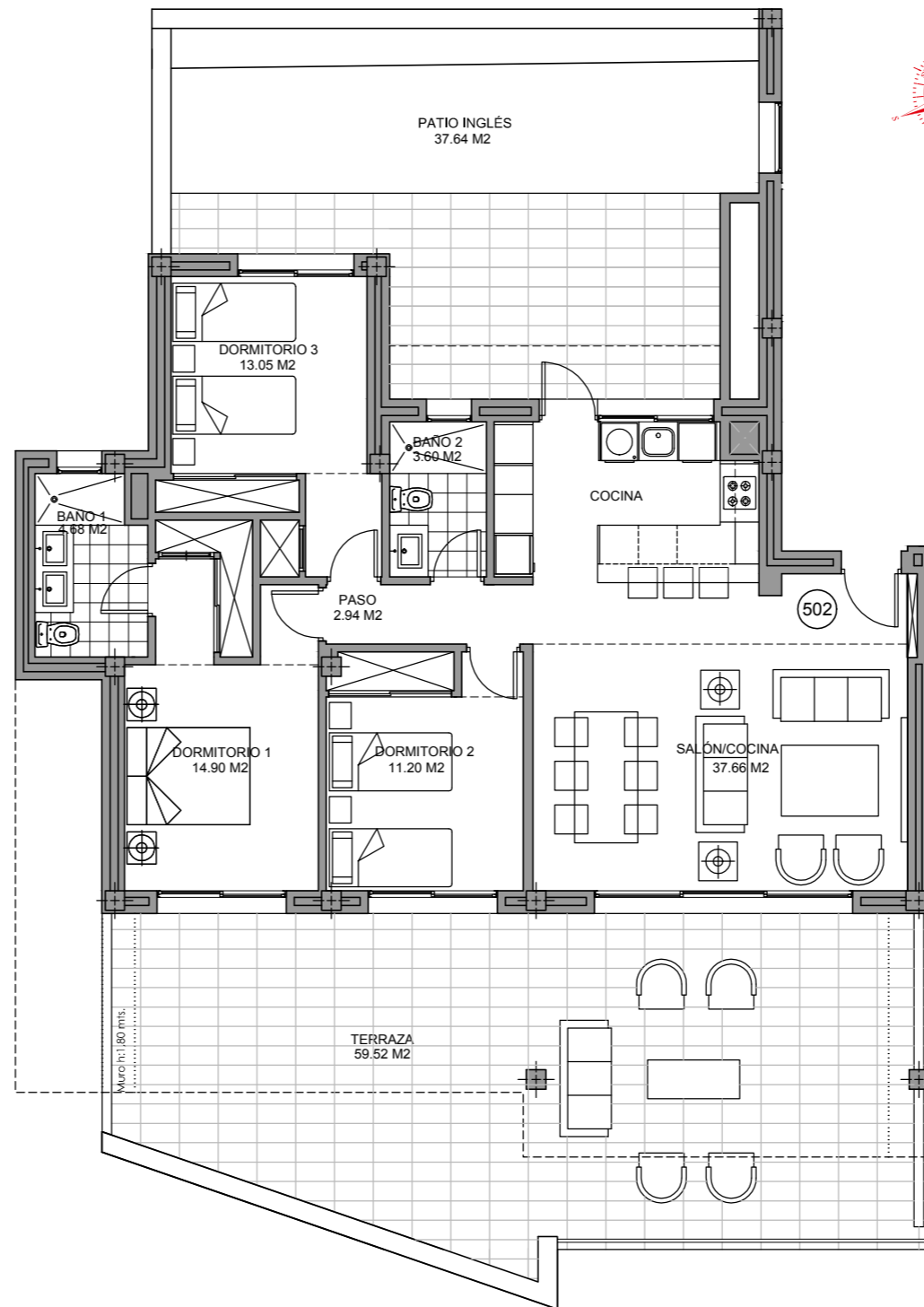
Planta Baja
