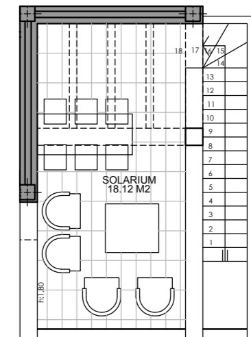
Planta Solarium
