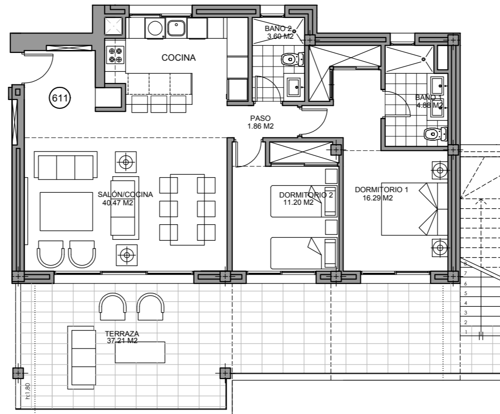
Planta Primera
