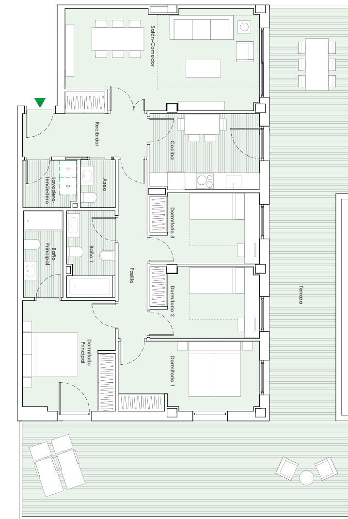
PISO 4 DORMITORIOS
