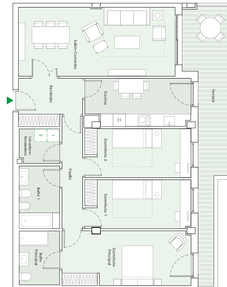
PISO 3 DORMITORIOS
