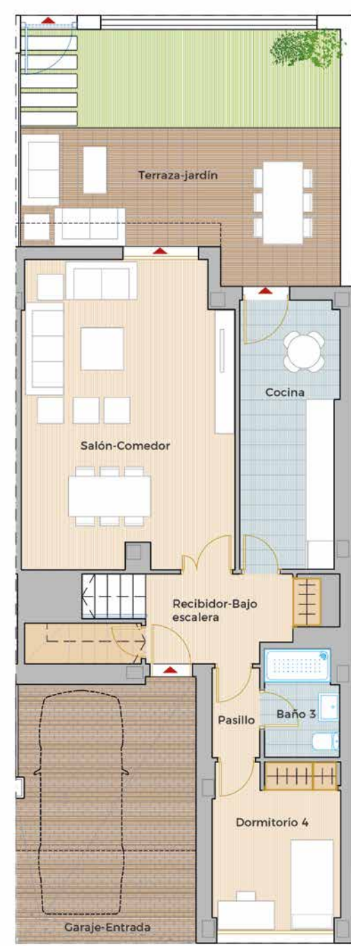
Planta baja
