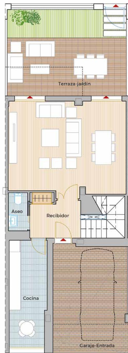
Planta baja
