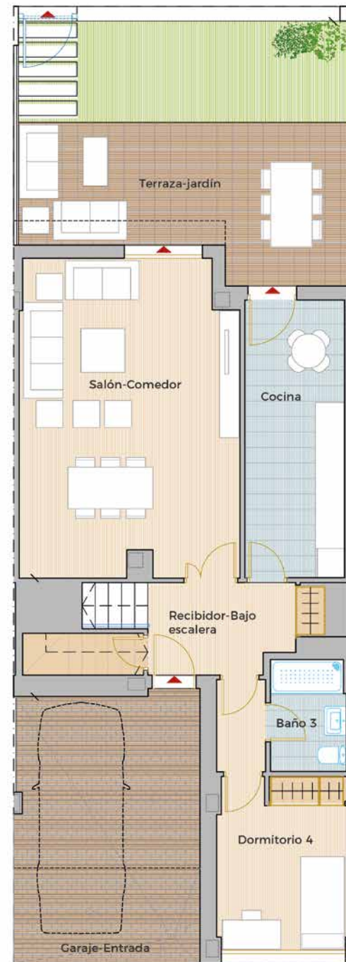
Planta baja
