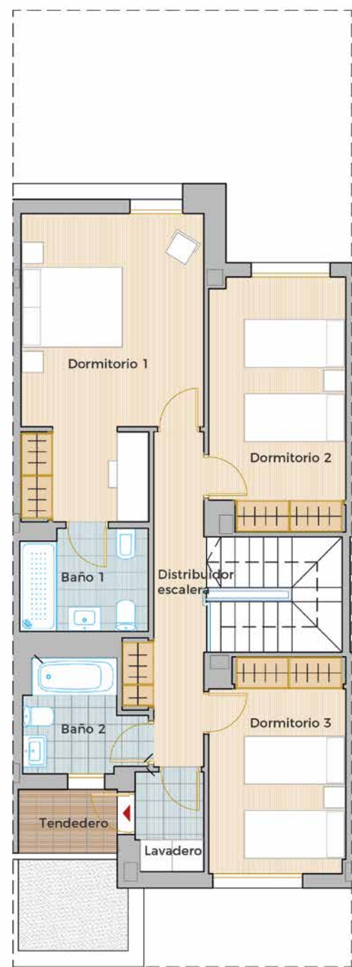
Planta primera
