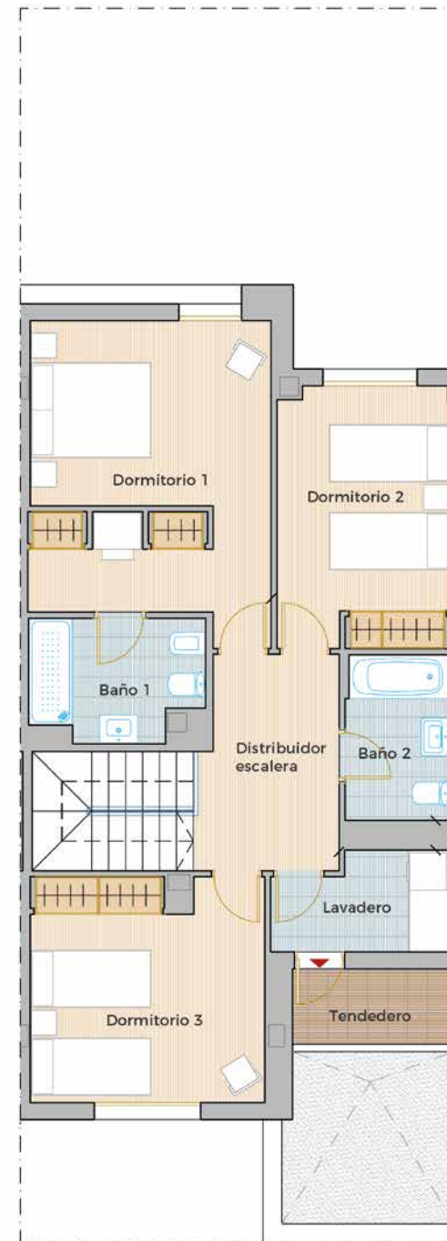
Planta primera
