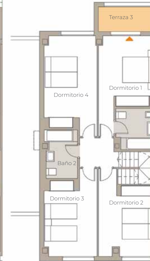
PLANTA PRIMERA
