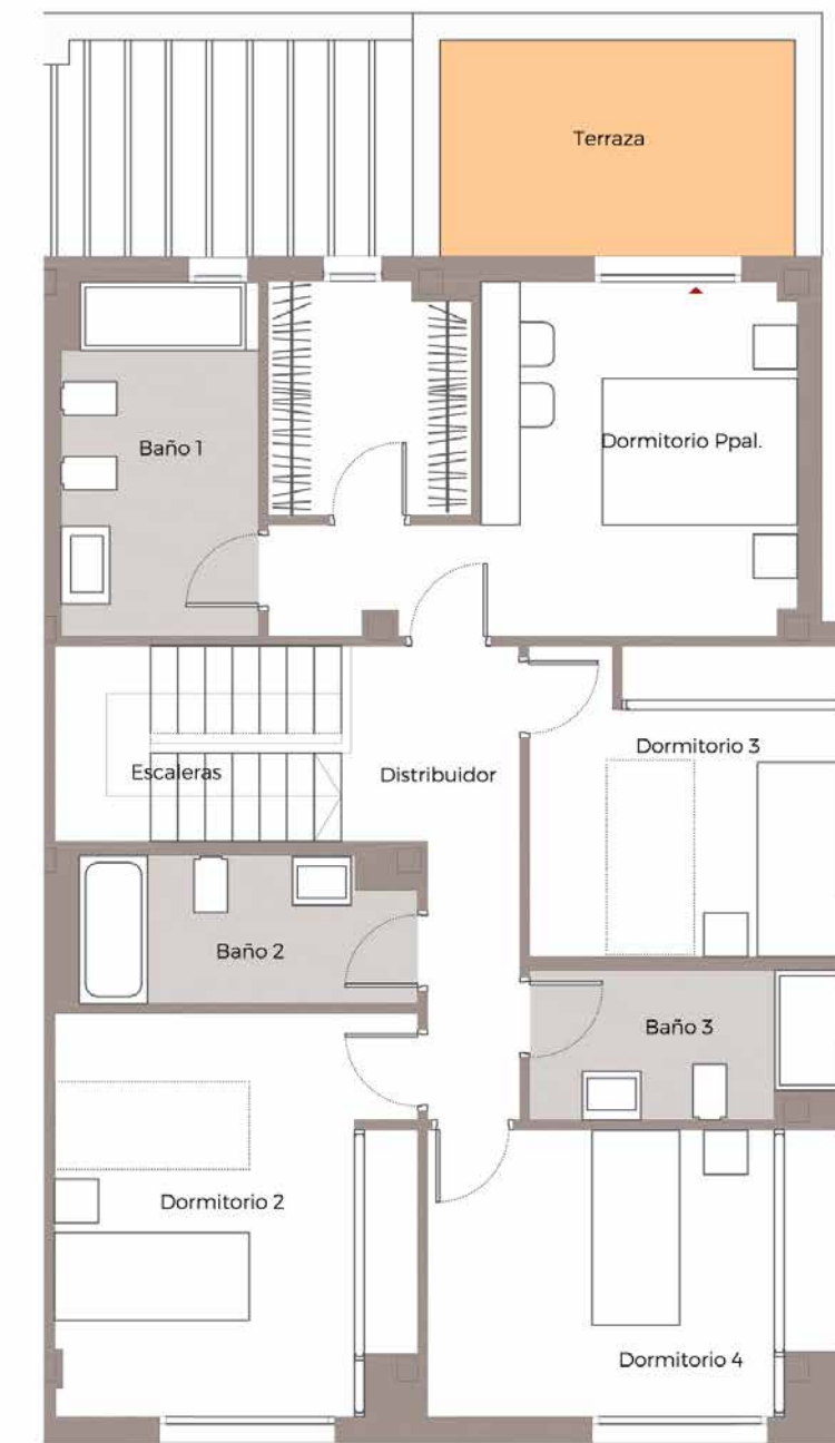
PLANTA PRIMERA
