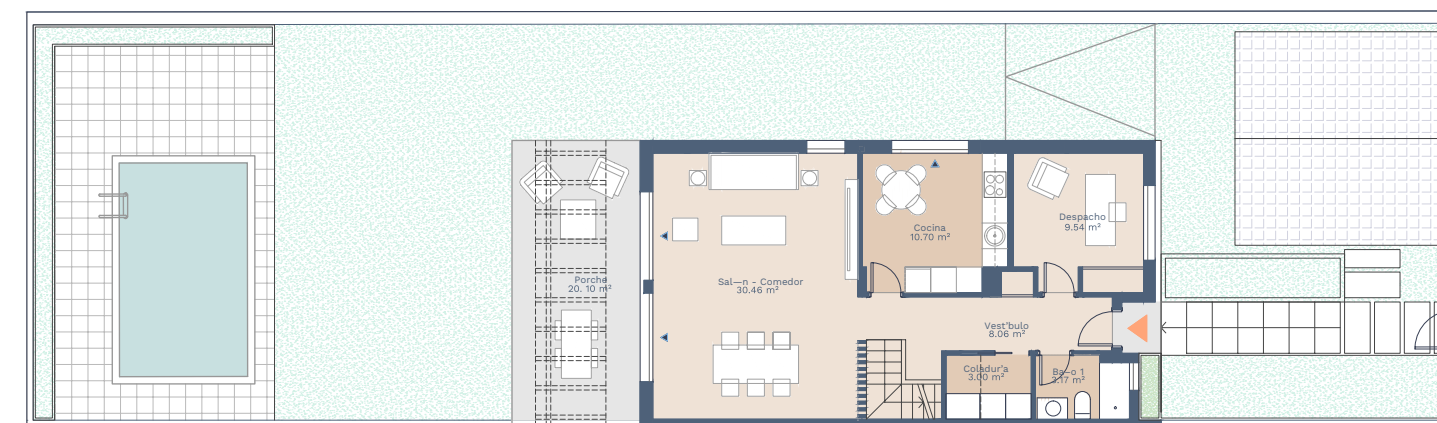
Planta Baja
