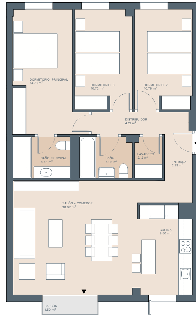
Bloque Oeste Esc 04 P02 y P04 - B
