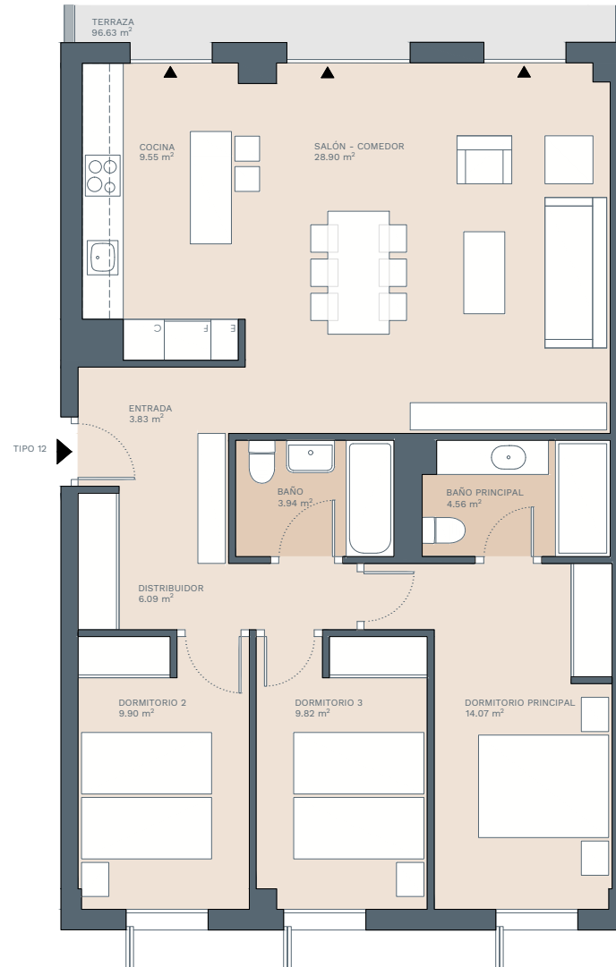
Bloque Oeste Esc 03 P01 - A
