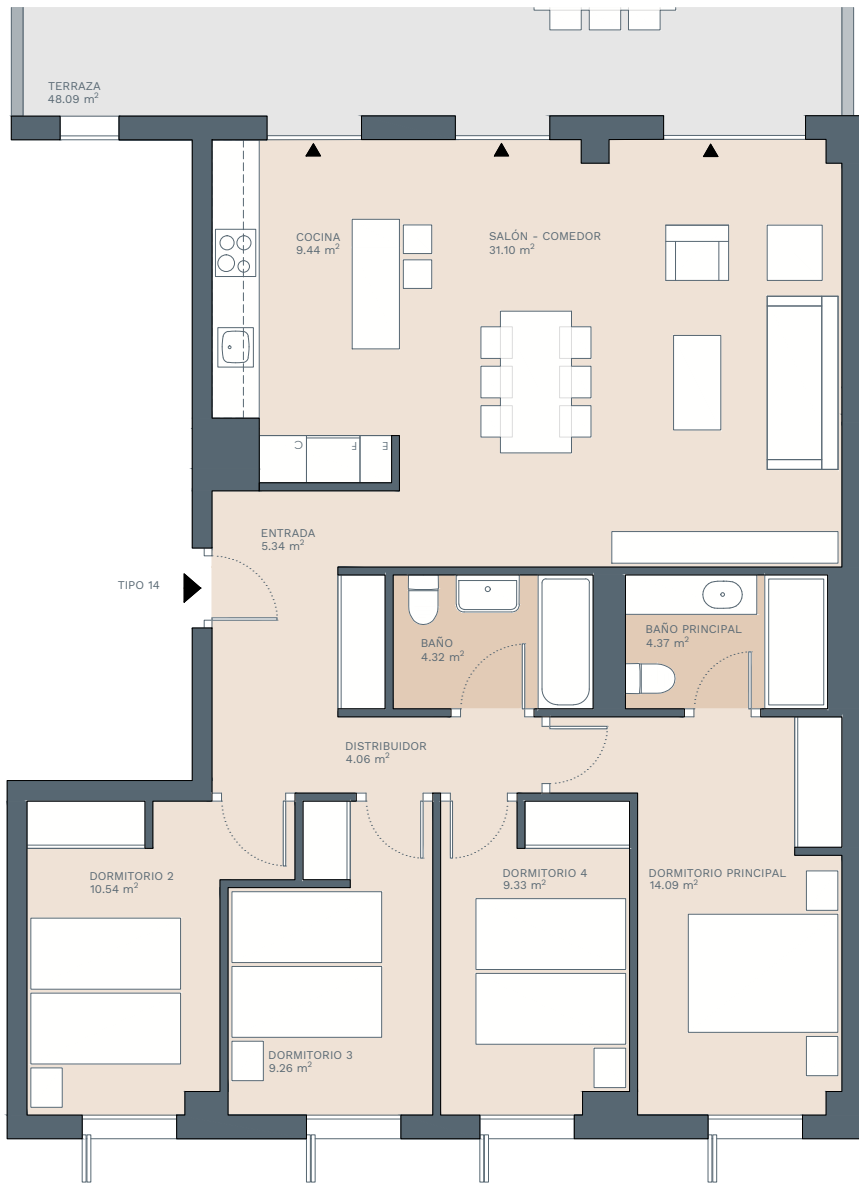
Bloque Oeste Esc 04 P01 - A
