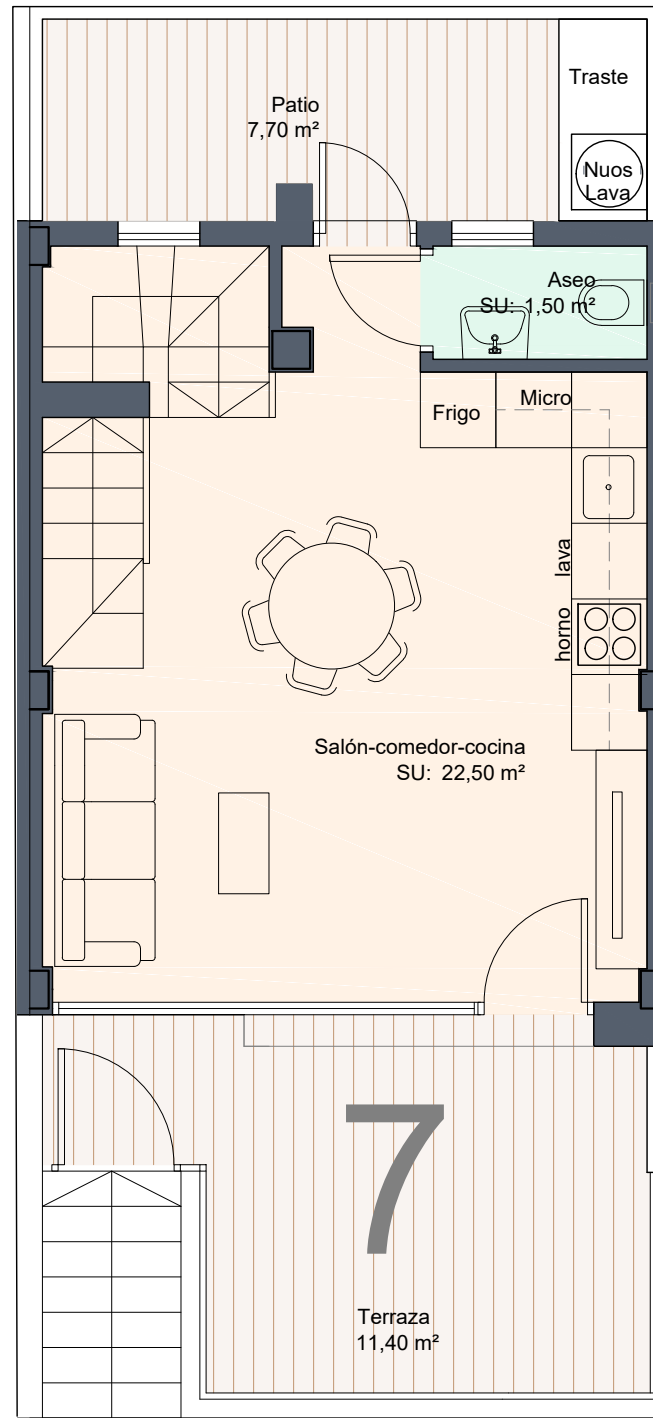
PLANTA BAJA
