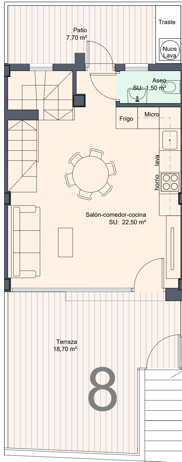
PLANTA BAJA
