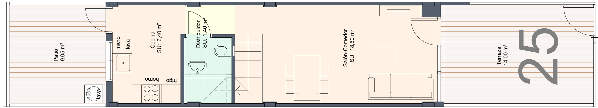
PLANTA BAJA
