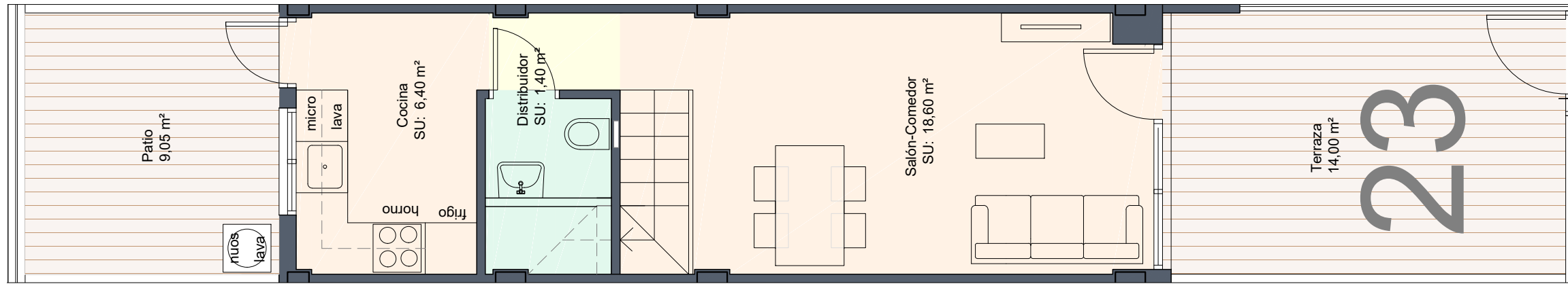
PLANTA BAJA
