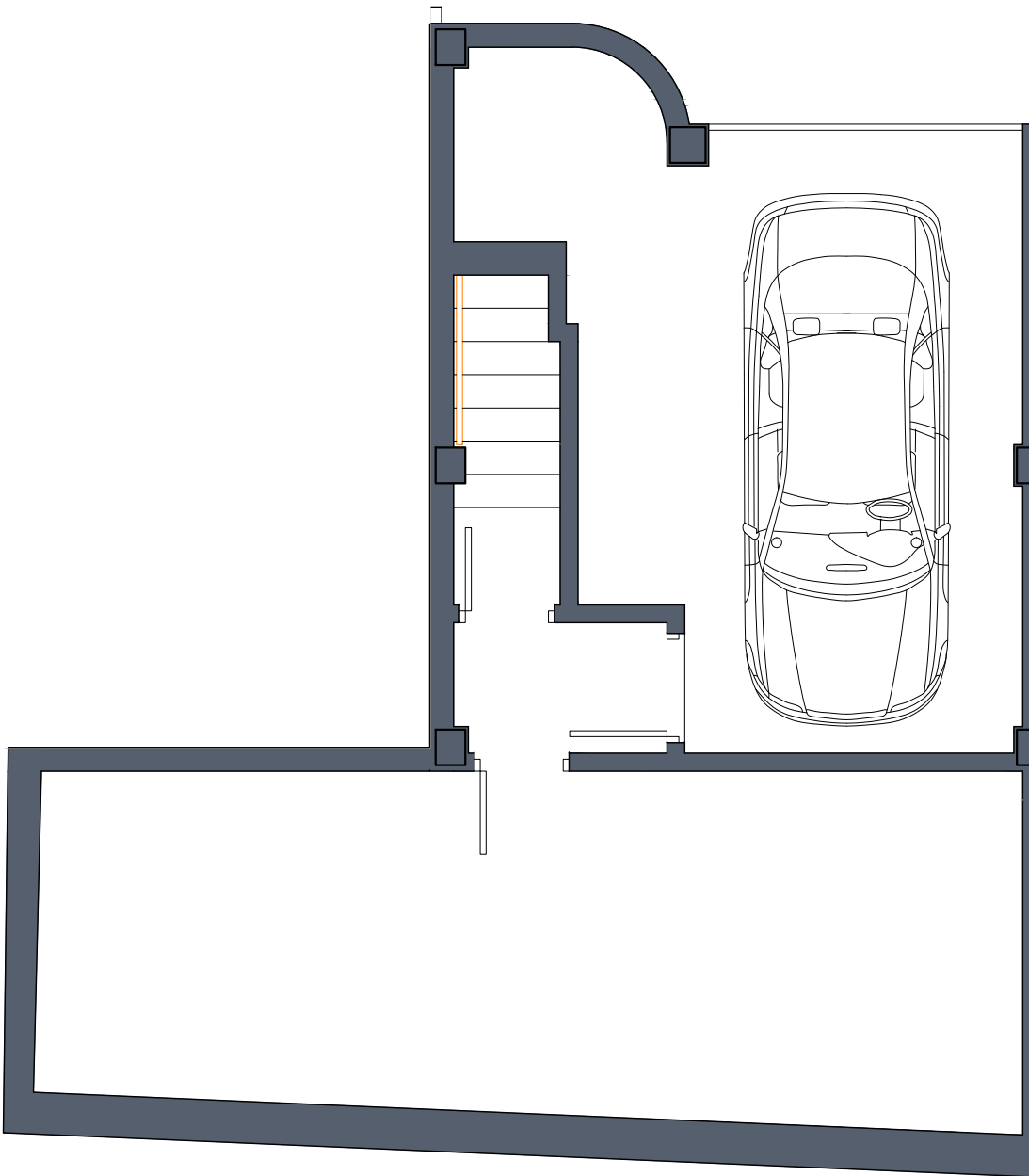
PLANTA SÓTANO
