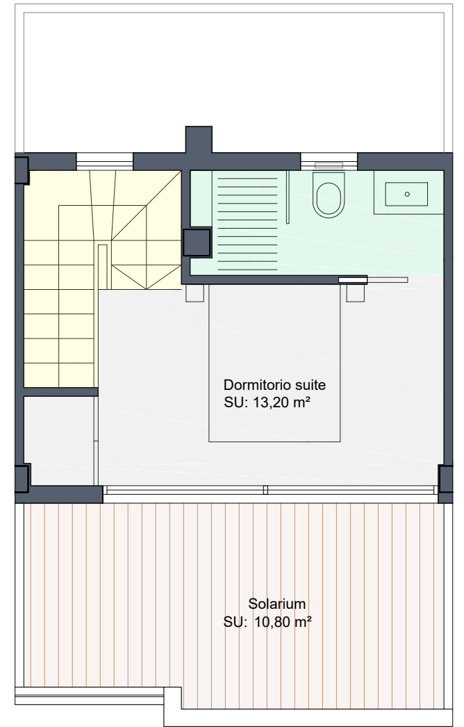
PLANTA SEGUNDA
