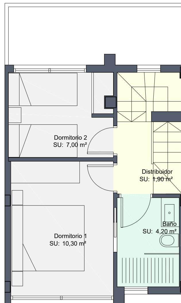
PLANTA PRIMERA
