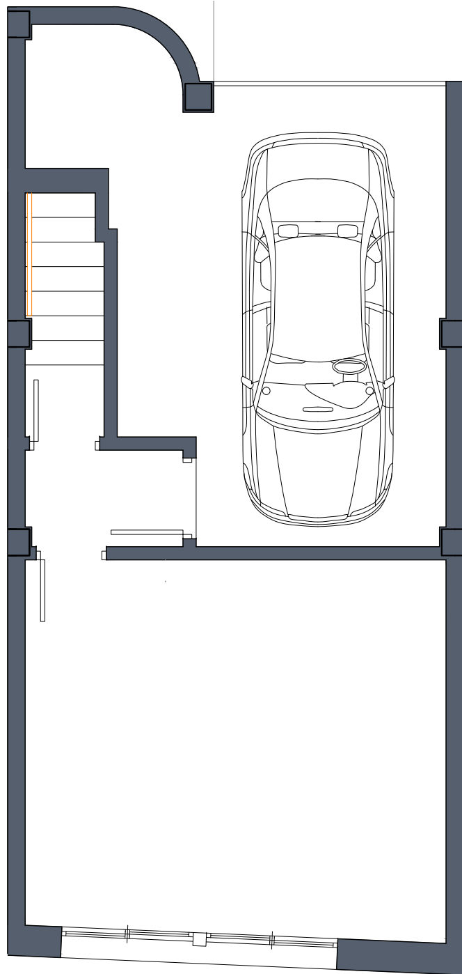
PLANTA SÓTANO
