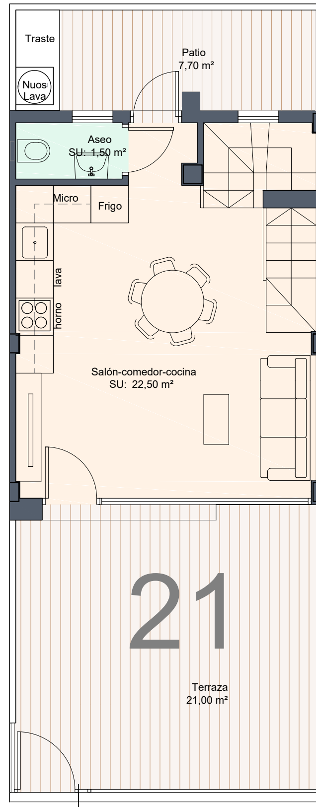
PLANTA BAJA
