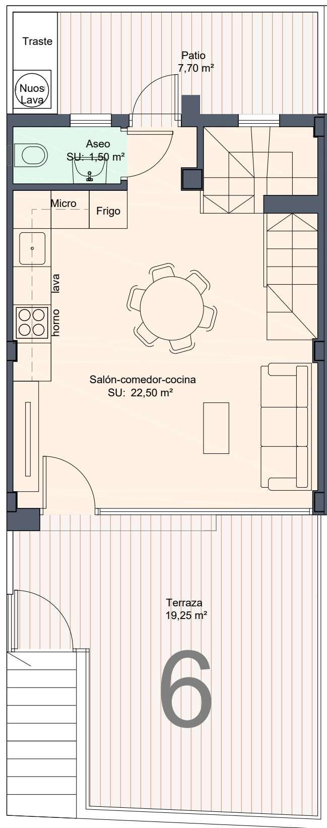
PLANTA BAJA
