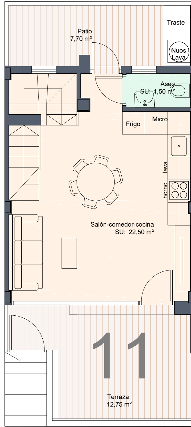
PLANTA BAJA
