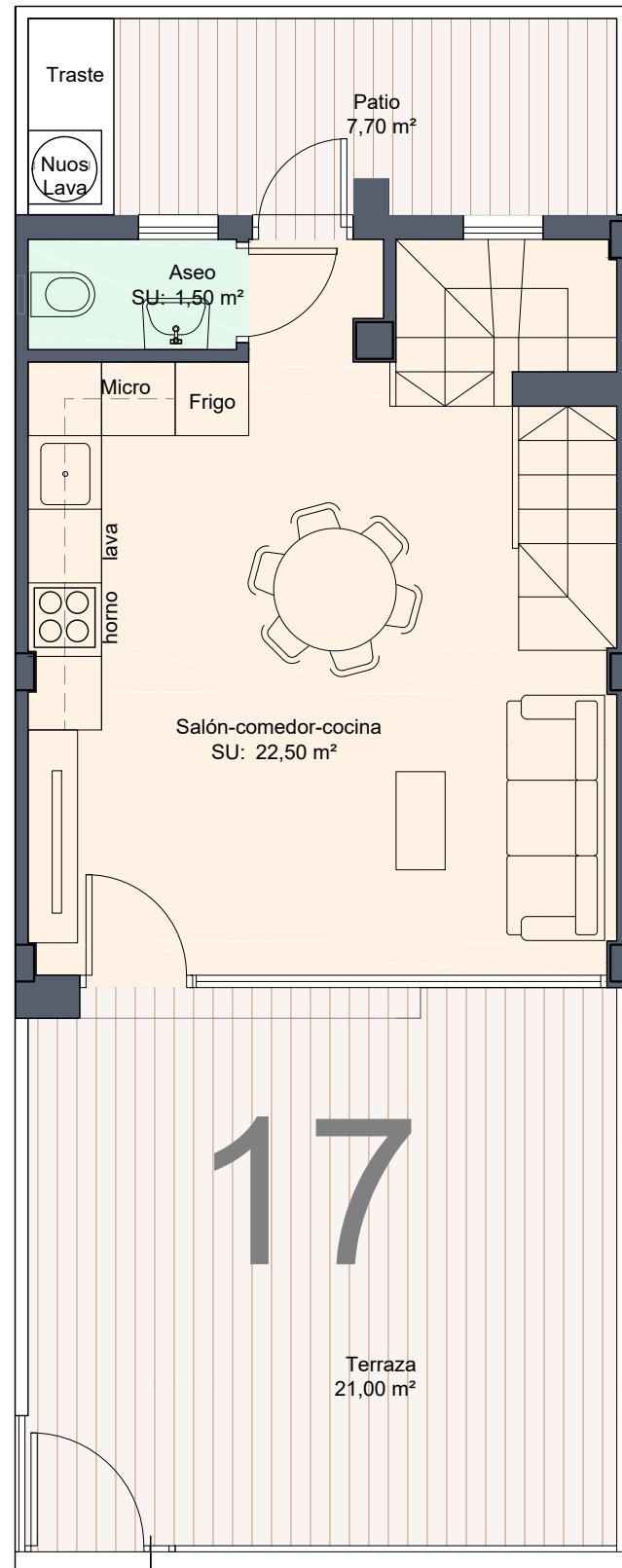
PLANTA BAJA
