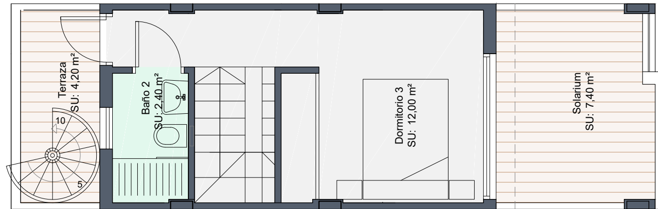
PLANTA SEGUNDA
