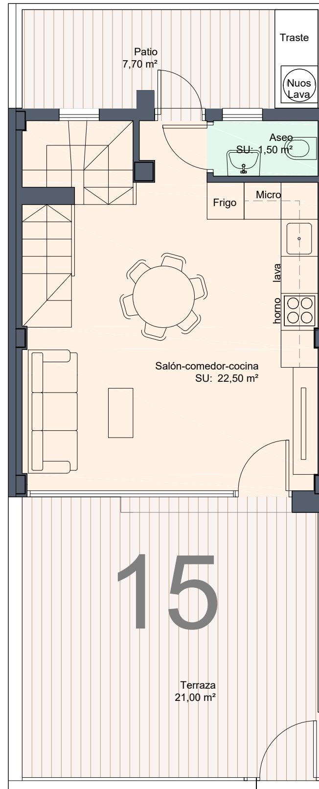
PLANTA BAJA
