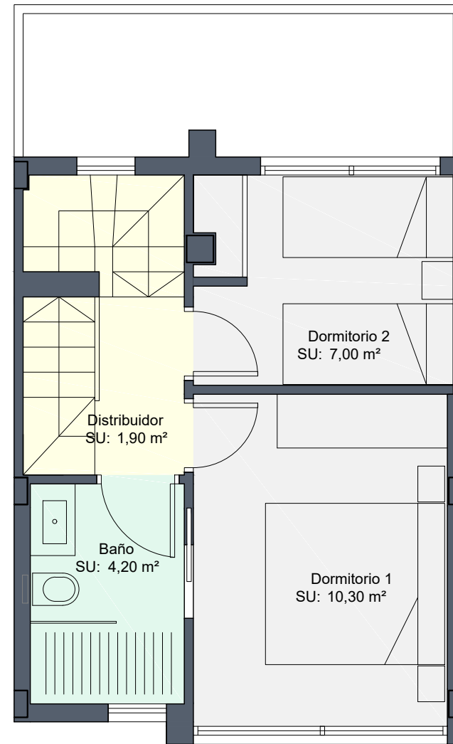
PLANTA PRIMERA
