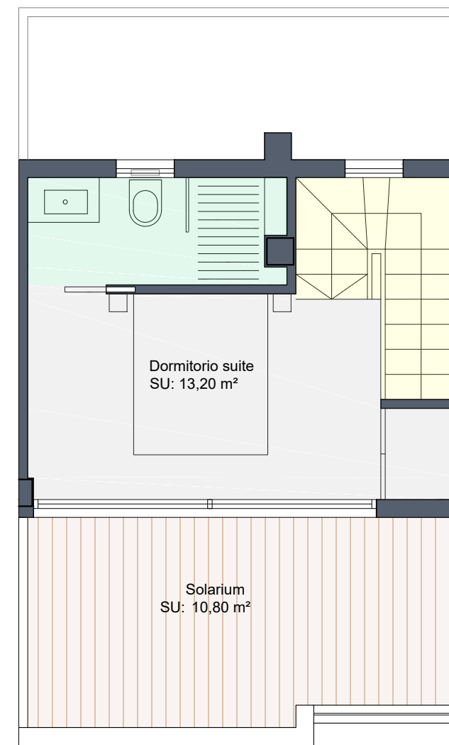
PLANTA SEGUNDA
