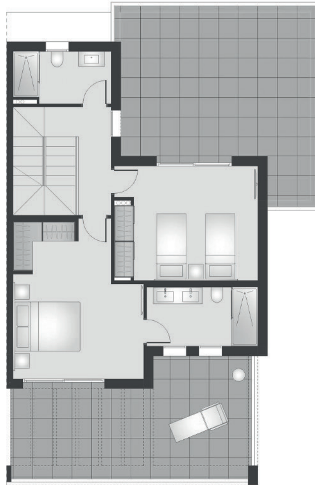
PLANTA SEGUNDA / SECOND FLOOR
