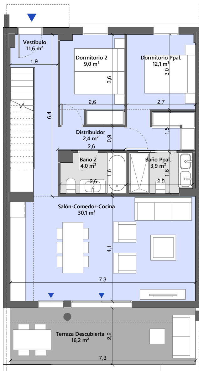
PLANTA BAJA
