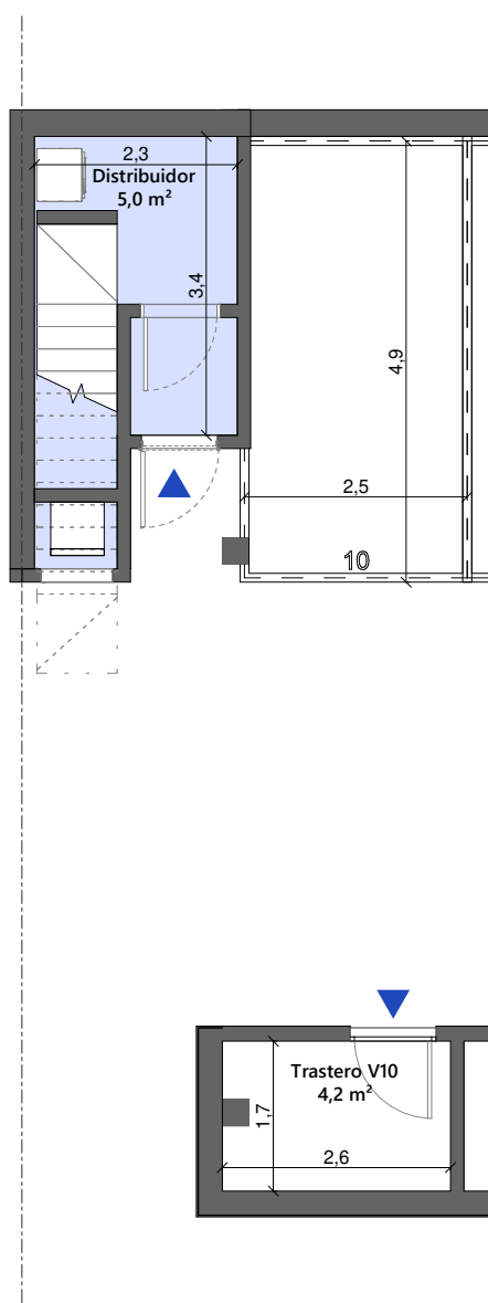
PLANTA SOTANO
