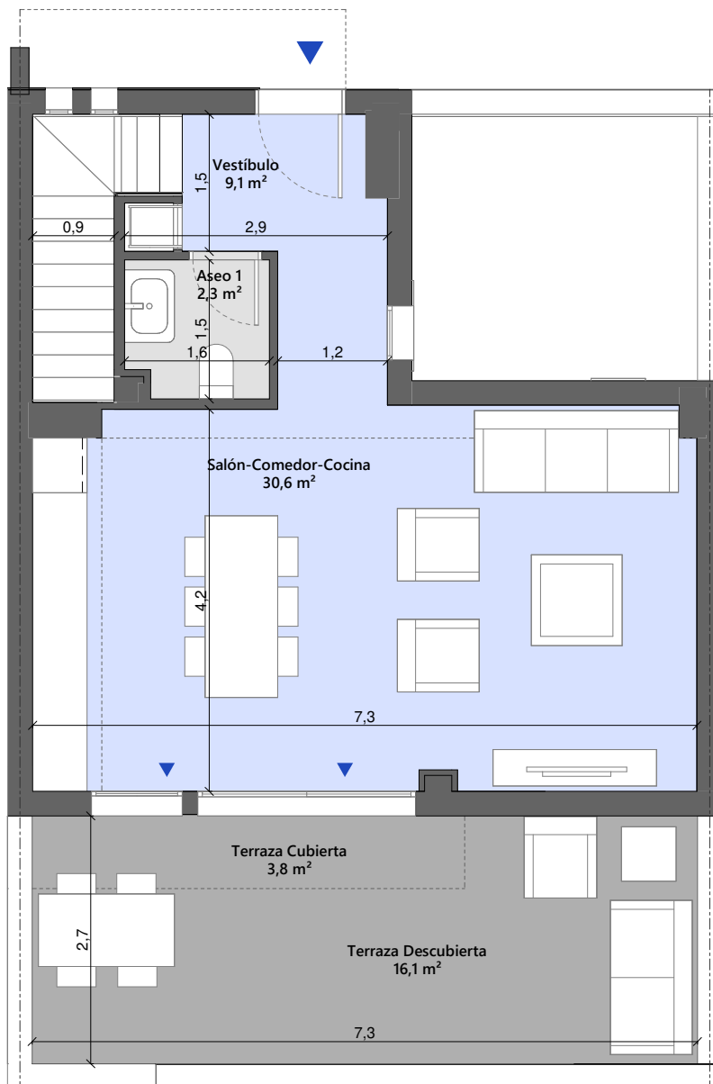
PLANTA BAJA
